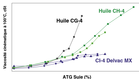
Test de moteur Mack T-8 (E)
